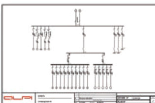
Einlinien-Schemadarstellung
